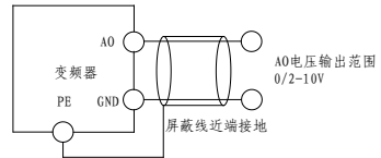
图 2-9 模拟输出端子配线图
