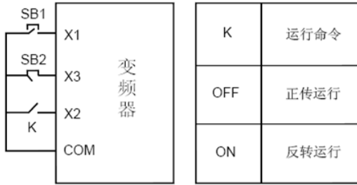
图5-2-4 三线式控制模式2
