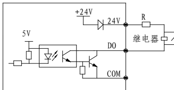
图 2-13 多功能输出端子开关量输出接线方式1
