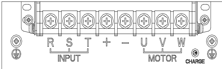
图 2-4 3PH 380V 18.5-37kW 主回路端子接线
