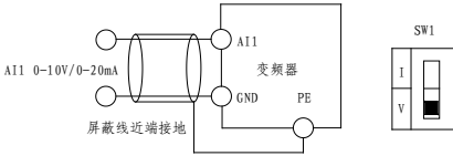
图 2-8 模拟输入端子配线图
