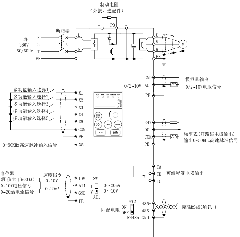
图 2-15 接线图
