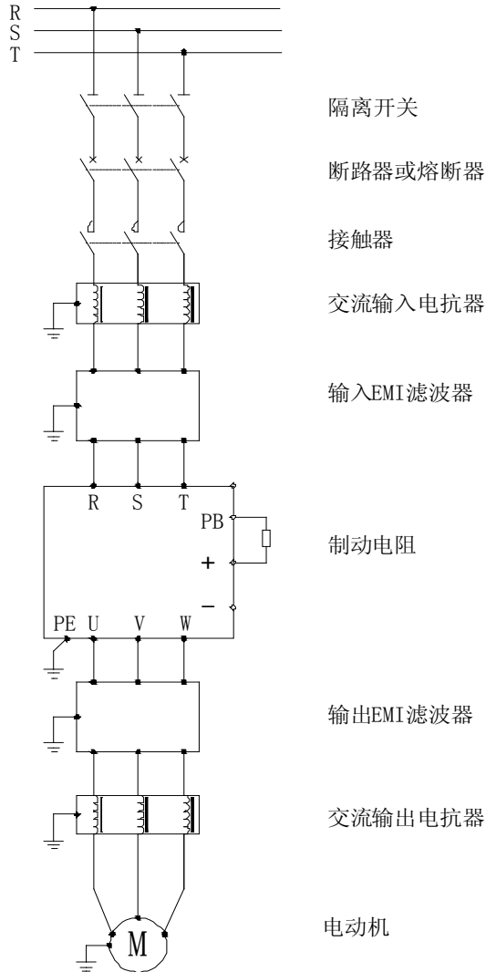
图 7-1 3R75GB-3022GB 外围设备连接图
