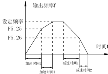
图5-5-6 加减速时间切换示意图
