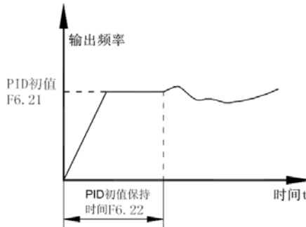
图5-6-3 PID初值功能示意图
