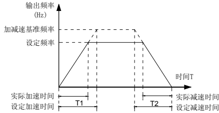
图 5-0-2 加减速时间示意图
