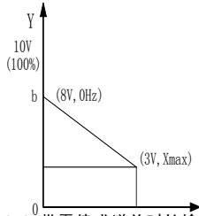
图5-3-2 带零偏或增益时的输出示意图(电压型)
