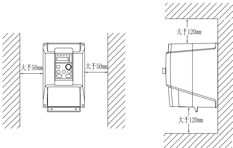
图 2-2 安装方向和空间
