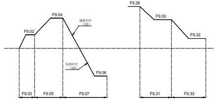
图5-8-1 简易PLC示意图
