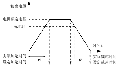
图5-9-3 V/F 分离示意图
