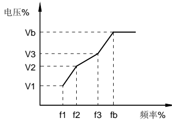
V1-V3: 多段速V/F第1-3段电压百分比 F1-F3: 多段速V/F第1-3段频率百分比 Vb: 电机额定电压, Fb: 电机额定运行频率
