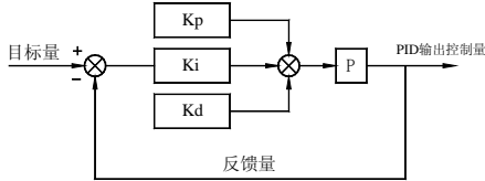
图5-6-1 过程PID 原理框图
