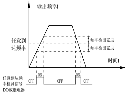
图5-5-7 任意到达频率检测示意图
