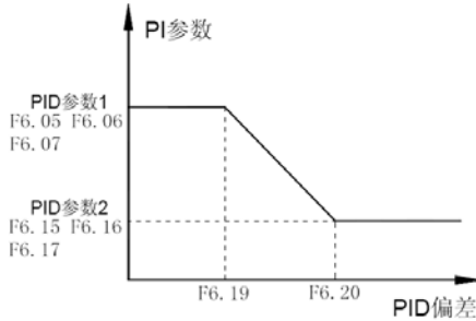
图5-6-2 PID 参数切换图
