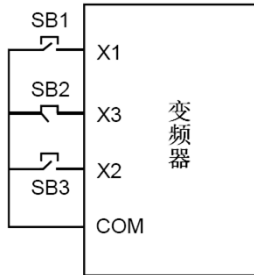
图5-2-3 三线式控制模式1
