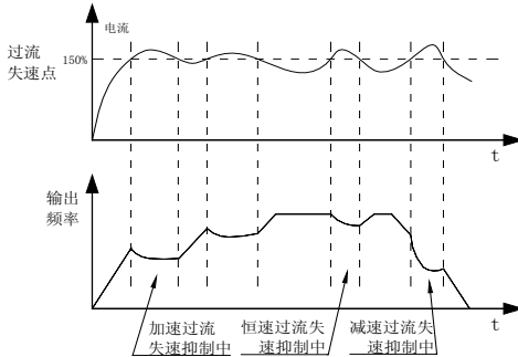
图5-9-6 过流失速动作示意图
