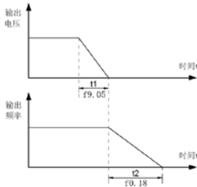
图5-9-5 V/F分离频率/电压先后下降示意图
