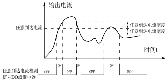
图5-5-10 任意到达频率检测示意图
