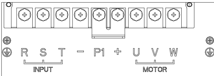
图 2-5 3PH 380V 37-160kW 主回路端子接线
