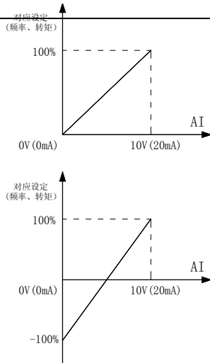
图5-2-5 模拟给定与设定量的对应关系
