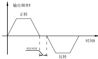
图5-5-2 正反转死区时间示意图
