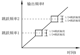
图5-5-1 跳跃频率示意图
