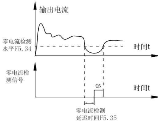
图5-5-8 零电流检测示意
