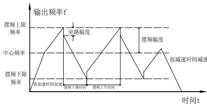
图5-7-1 摆频运行示意图
