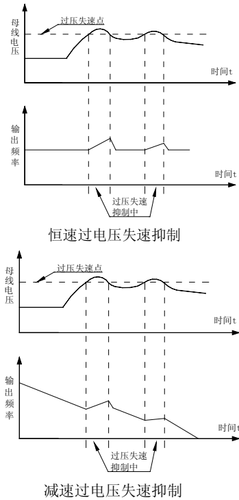
图5-9-8 过电压失速动作示意图
