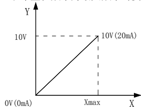
图5-3-1 无零偏或增益时的输出示意图
