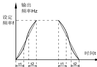
图5-4-1 静态S曲线示意图
