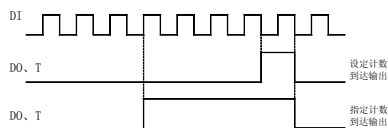
图 5-8-2 设定计数值和指定计数值示意图
