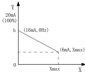
图5-3-3 带零偏或增益时的输出示意图(电流型)
