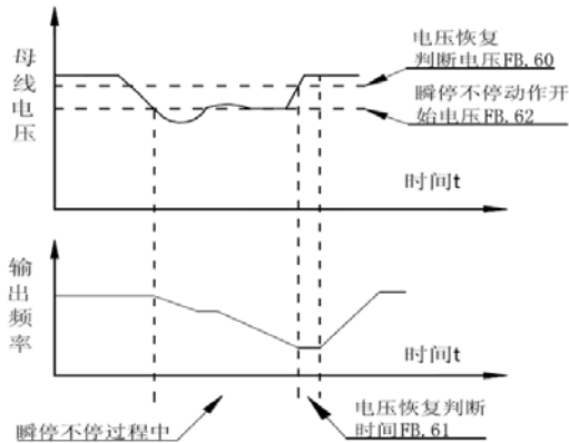
图5-B-2 瞬停不停过程示意图
