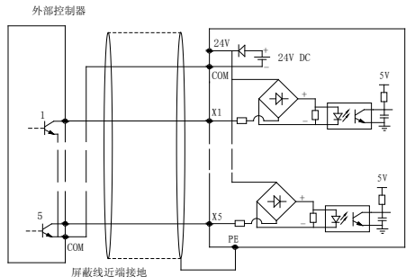
图2-12 输入多功能端子配线连接图
