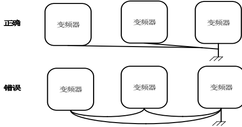
图 2-6 接地线连接方法
