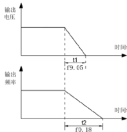
图5-9-4 V/F 分离输出电压/ 频率独立减至0
