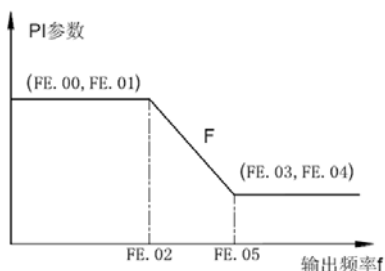
图5-E-1 PI参数示意图
