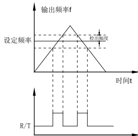
图5-5-4 频率到达检出幅值示意图
