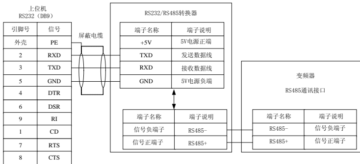
图 2-10 上位机与变频器接口接线图
