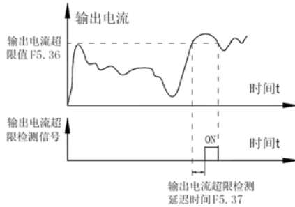
图5-5-9 输出电流超限检测示意图
