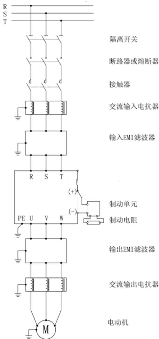
图 7-2 3030GB 及以上外围设备连接图
