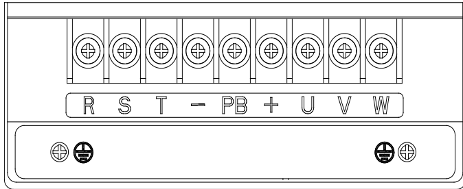
图 2-3 3PH 380V 4-15kW 主回路端子接线
