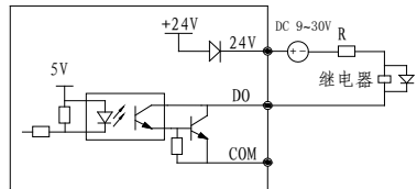
图 2-14 多功能输出端子开关量输出接线方式2
