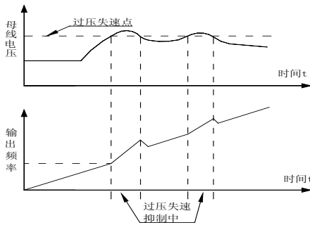
加速过电压失速抑制
