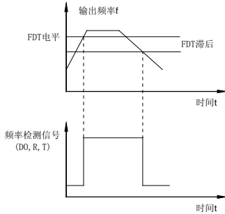
图5-5-3 FDT电平示意图
