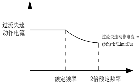
图5-9-7 倍速过流失速动作示意图
