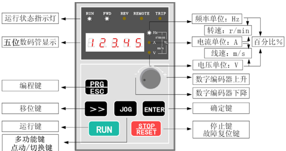
图 3-1 键盘布局与各部分名称
